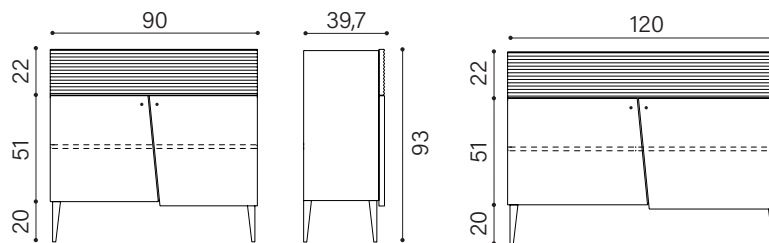
Consolle 2 ante battenti e cassetto / Consolle 2 hinged doors
